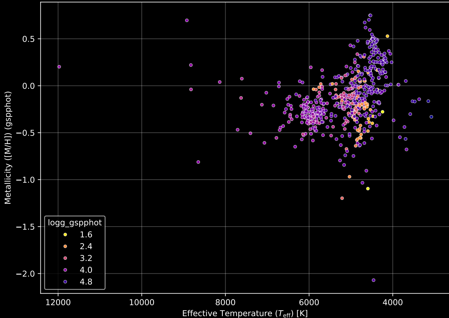
APOGEE DR17 Field: [M67] Stellar Population Parameters (n= 588)
